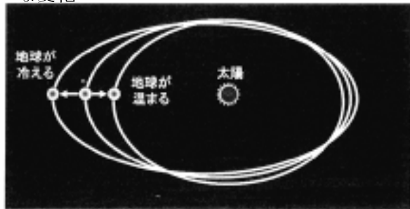
地球の軌道は約10万年の周期で、正円に近づいたり楕円になったりしている。この間、地球と太陽の距離は、100万km以上も変化する。
