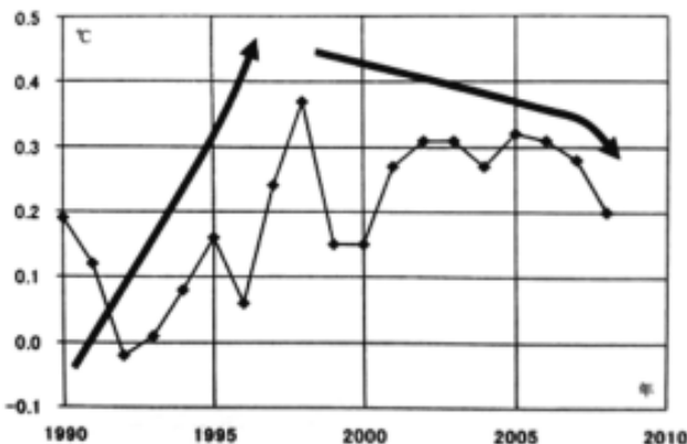
地球の気温は急上昇すると騒いできたが、CO2は激増しながら気温が上がらず、みな説明に困っている。2009年気象庁公表値より。
