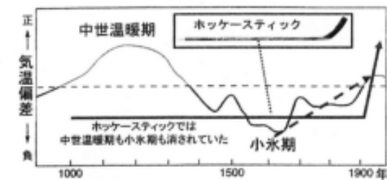
1990年のIPCC第1次報告書には正しく中世温暖期と小氷期が明示されていた
