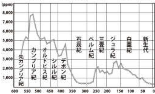
過去6億年の二酸化炭素 (CO2) 量の変化の推定例
